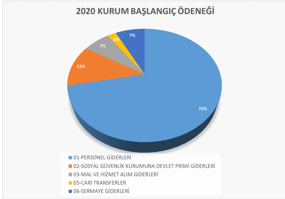
Grafik 1. 2020 Yılı KBÖ Ekonomik Sınıflandırmaya Göre Dağılımı
